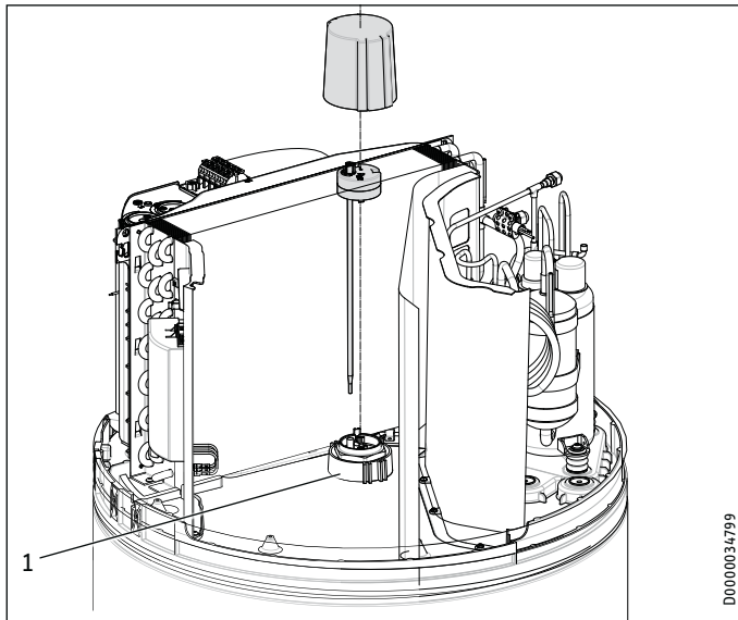
1 Calentador eléctrico de refuerzo con ánodo protector
